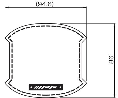
寸法図
