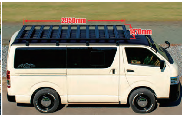
●EXR-03 EXPルーフラックtypeC ●サイズ：W.1470mm D.2950mm H.38.8mm(取付用レッグ除く)
